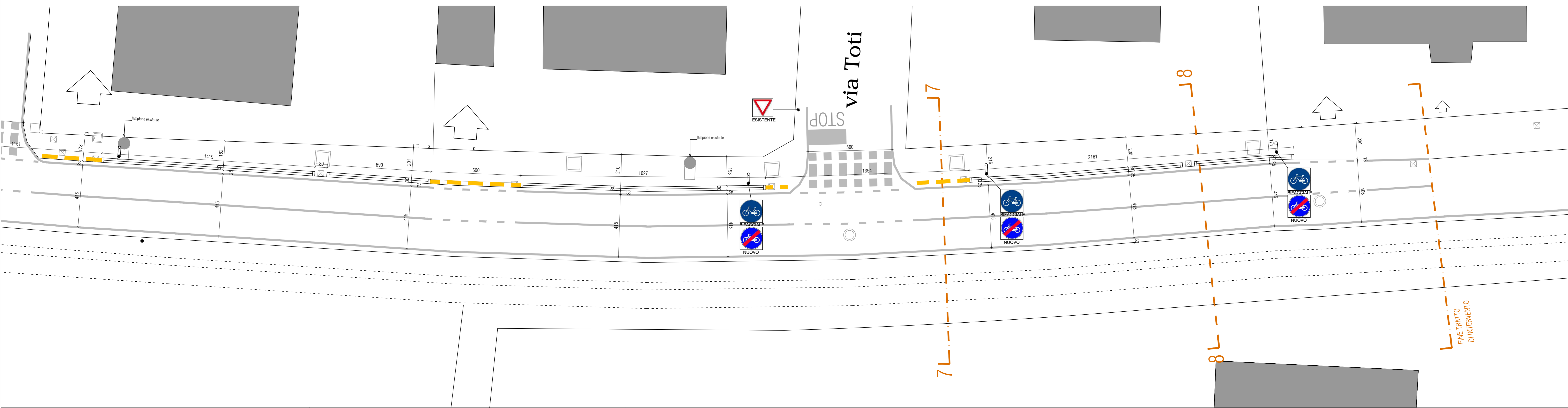
PLANIMETRIA DI PROGETTO QUOTATA DELLA SEDE STRADALE - TRATTO 7/7 Scala 1:100
